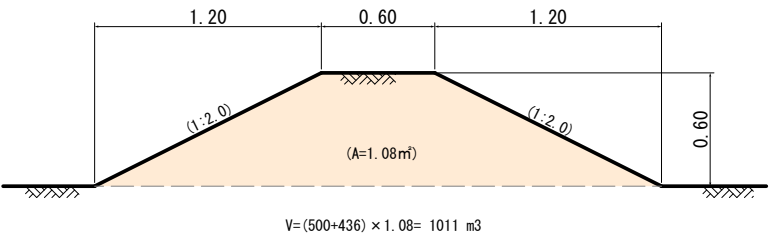
盛土小堤
